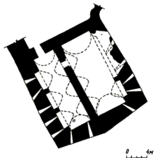
Grundriss Südturm
