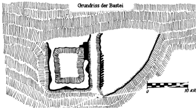
Grundriss der Bastei
